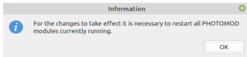
Fig. 12. Information message
