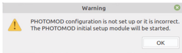
Fig. 7. Information message
