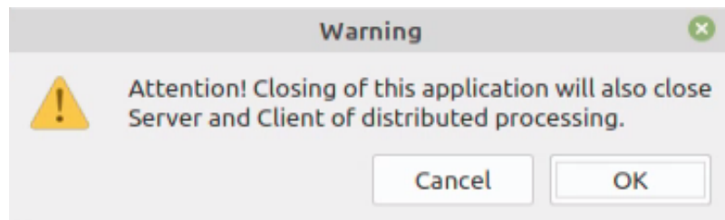
Fig. 21. Information message
