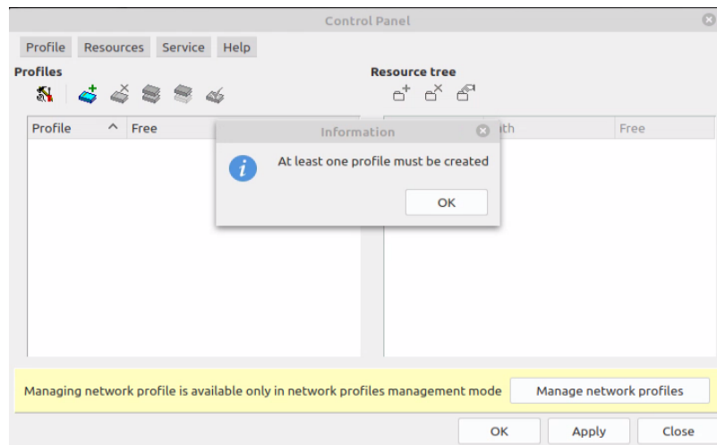
Fig. 9. Information message
