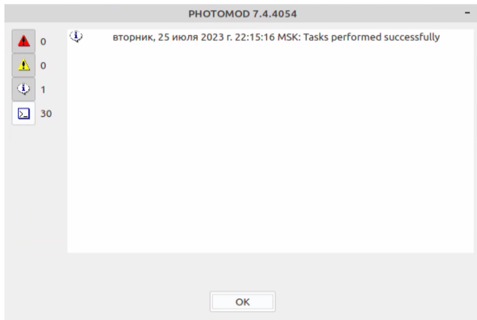
Fig. 20. Information message
