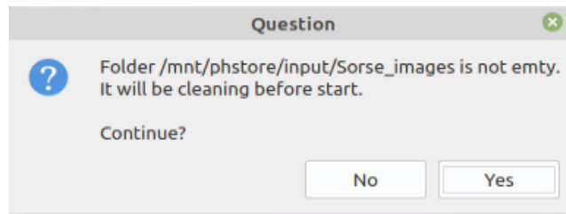
Fig. 18. Information message
