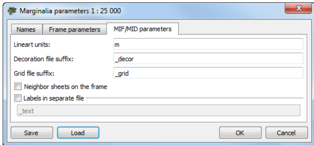
Fig. C.26. Marginalia parameters
