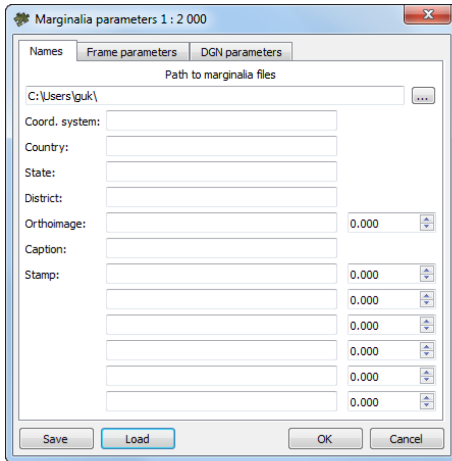
Fig. C.1. Marginalia parameters
