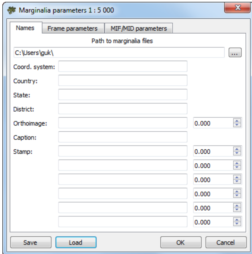
Fig. C.12. Marginalia parameters
