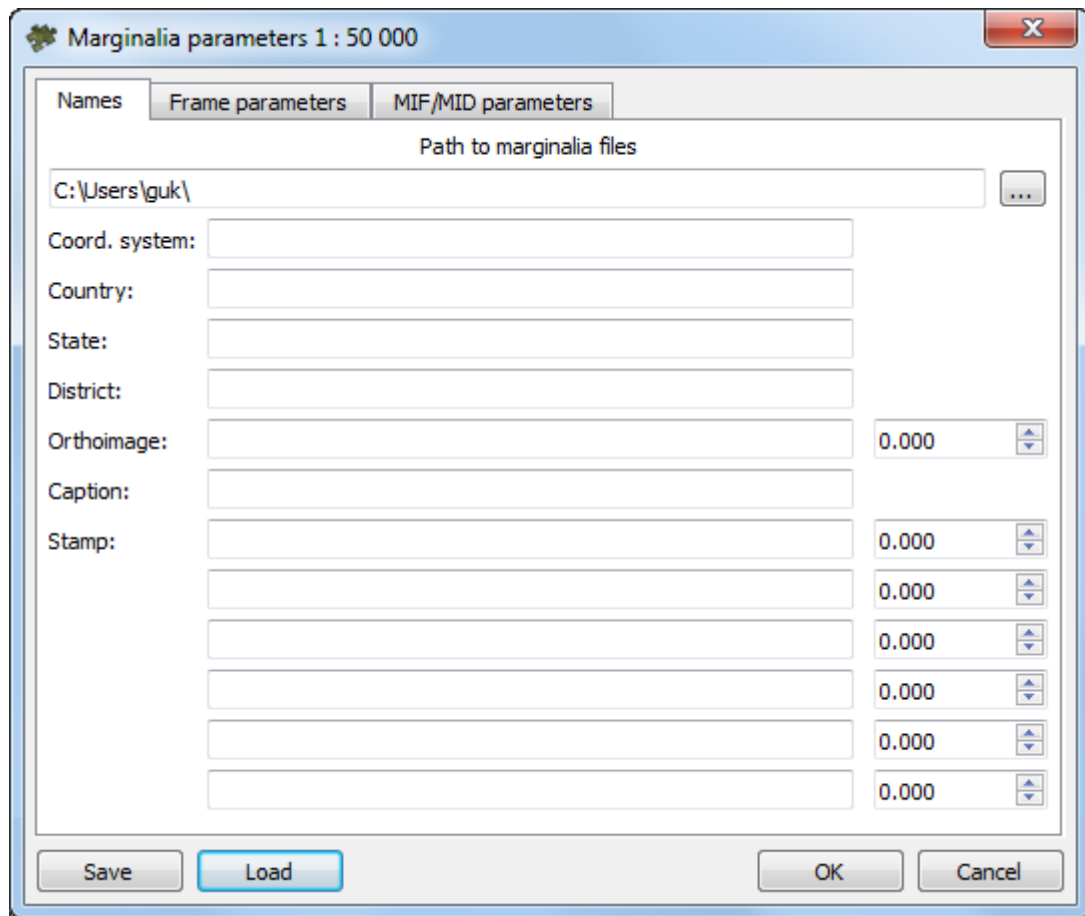
Fig. C.30. Marginalia parameters
