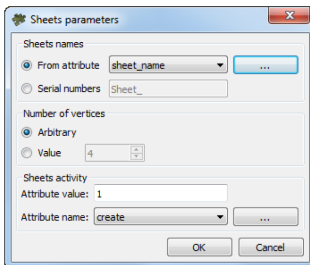
Fig. 58. Sheets parameters
