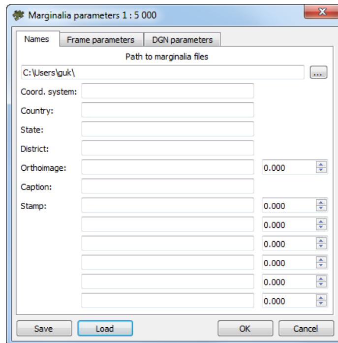
Fig. C.9. Marginalia parameters
