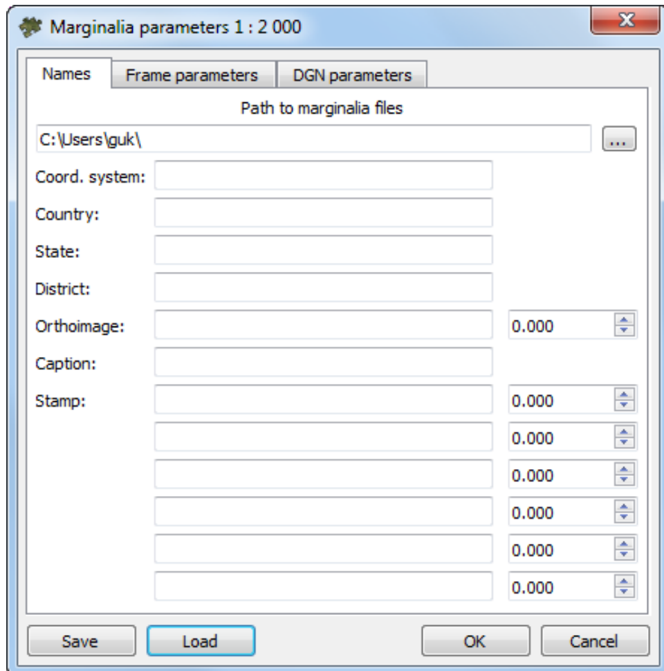
Fig. C.3. Marginalia parameters
