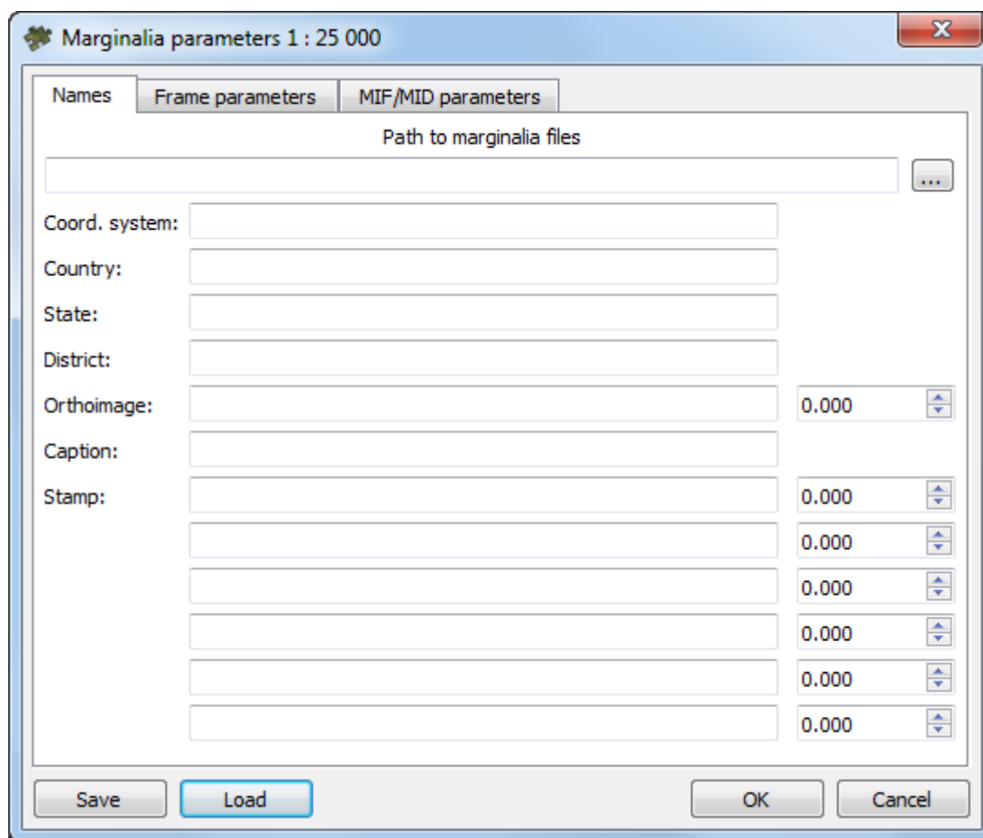
Fig. C.24. Marginalia parameters
