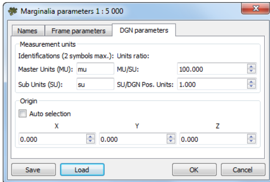
Fig. C.11. Marginalia parameters
