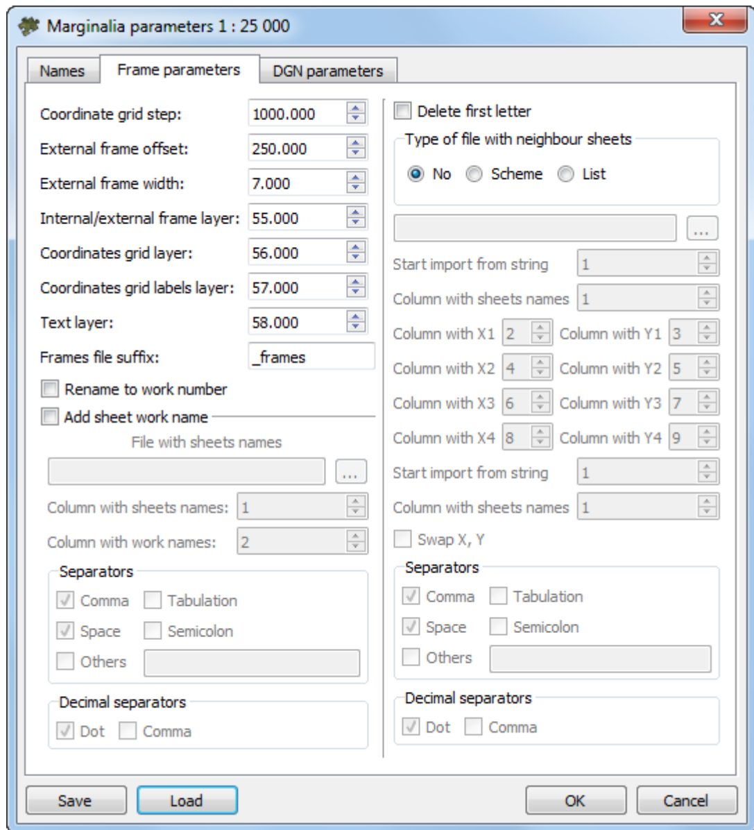
Fig. C.22. Marginalia parameters
