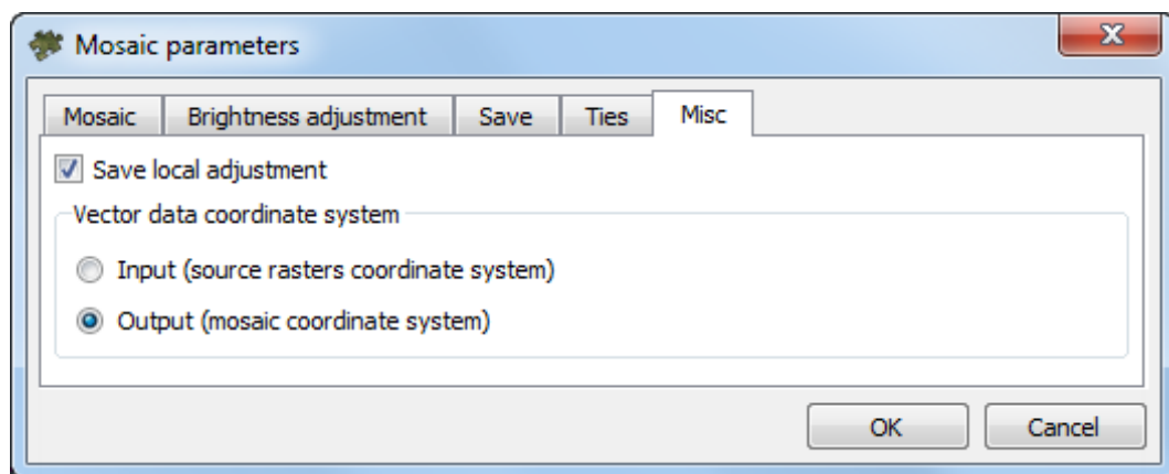
Fig. 70. Additional parameters
