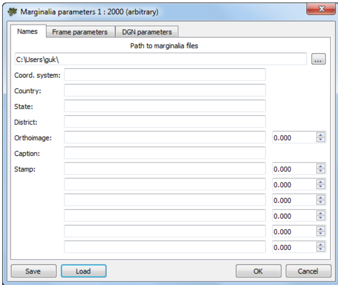
Fig. C.33. Marginalia parameters
