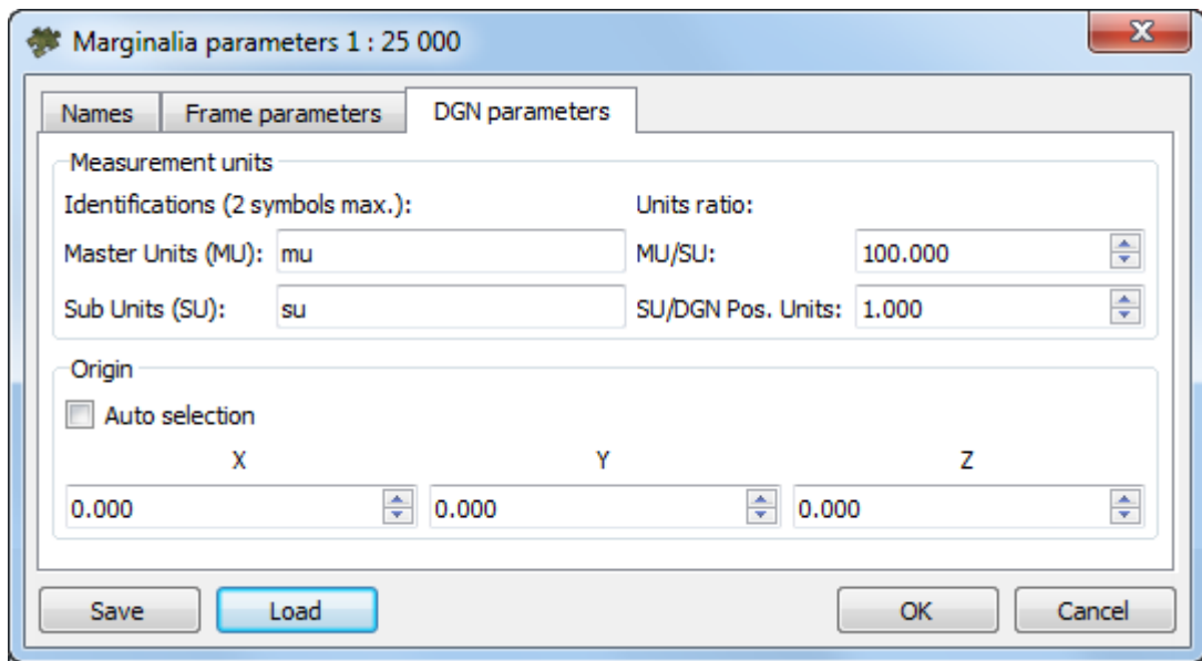
Fig. C.23. Marginalia parameters
