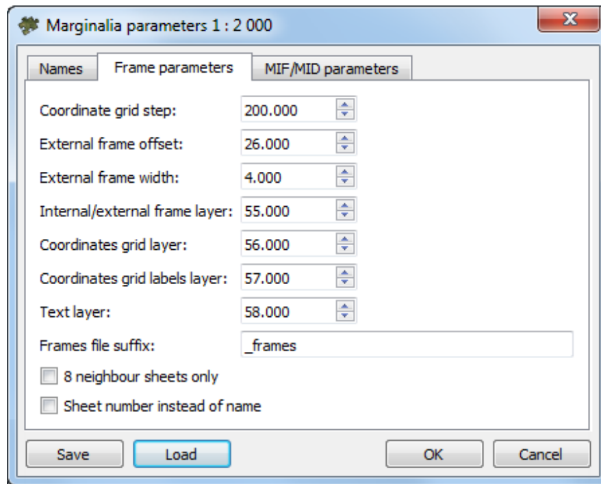
Fig. C.7. Marginalia parameters
