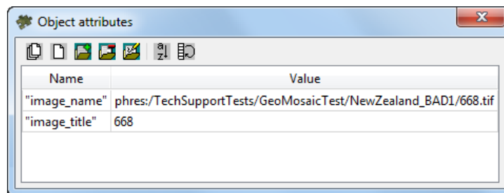
Fig. 27. Cutlines attributes
