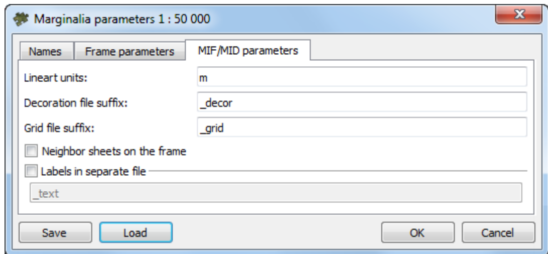
Fig. C.32. Marginalia parameters
