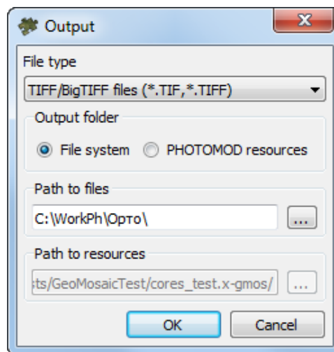
Fig. 71. Output parameters
