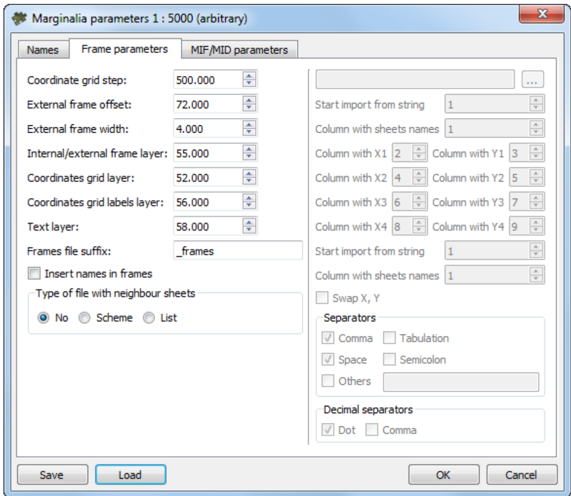
Fig. C.34. Marginalia parameters
