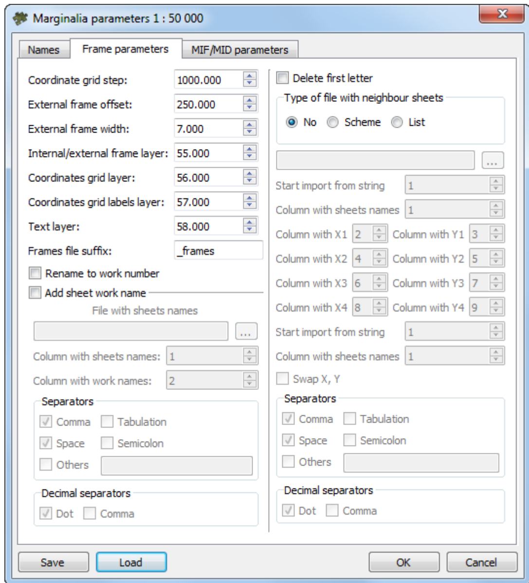
Fig. C.31. Marginalia parameters
