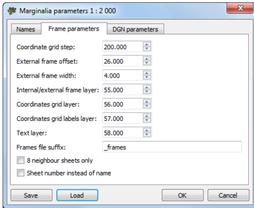
Fig. C.4. Marginalia parameters
