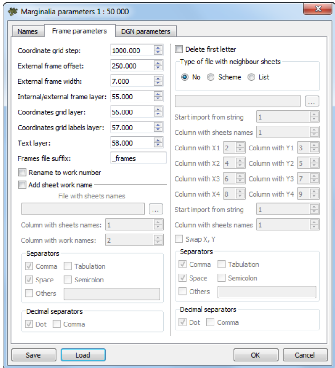
Fig. C.28. Marginalia parameters
