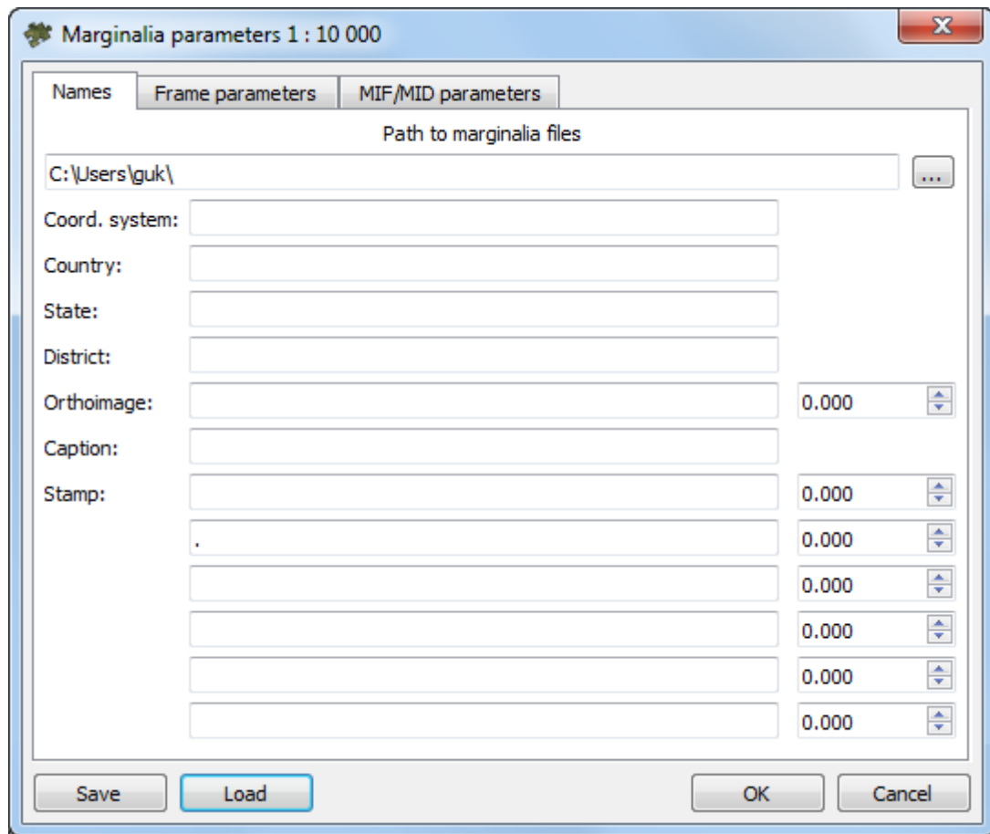
Fig. C.18. Marginalia parameters
