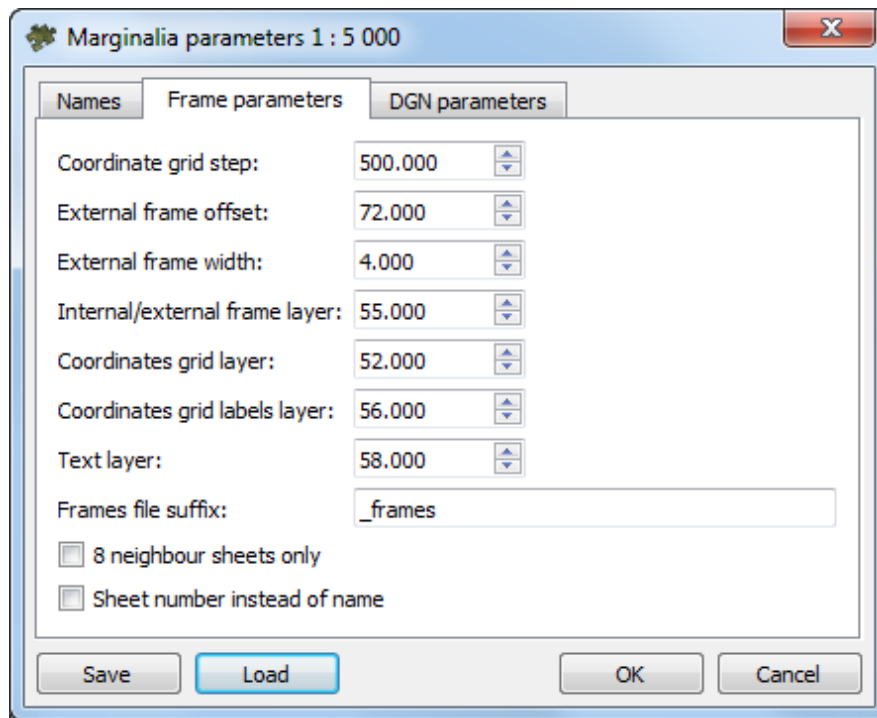
Fig. C.10. Marginalia parameters
