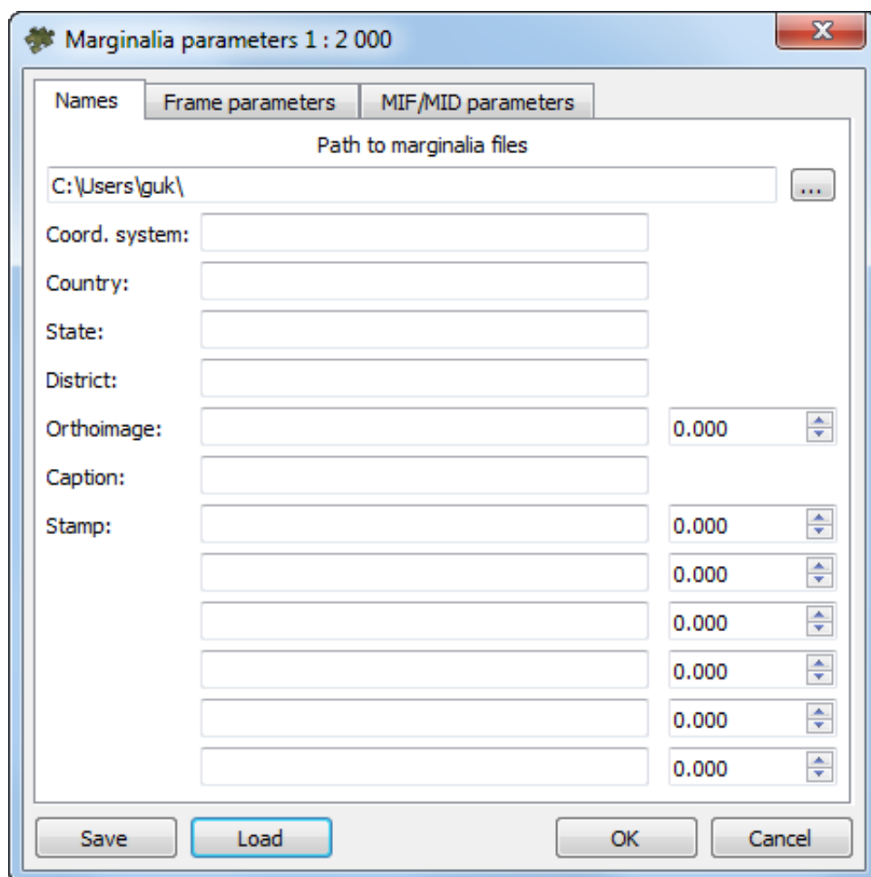
Fig. C.6. Marginalia parameters
