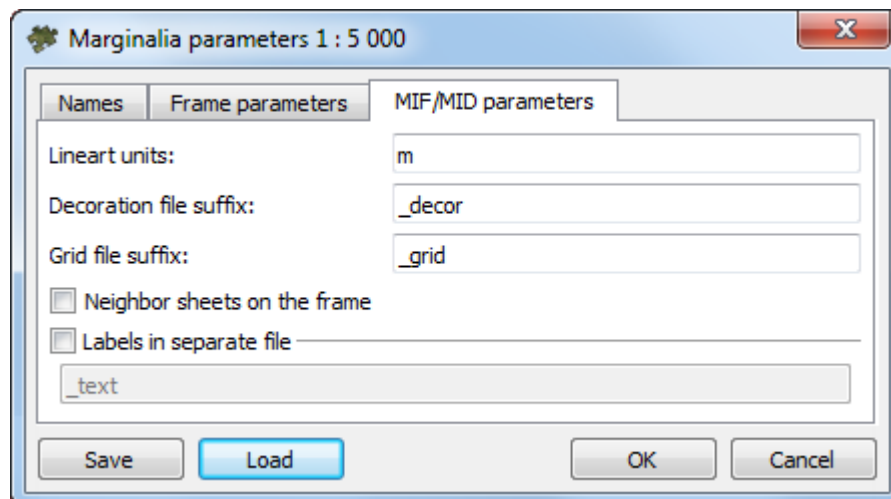
Fig. C.14. Marginalia parameters
