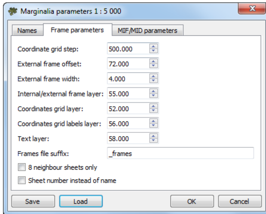
Fig. C.13. Marginalia parameters
