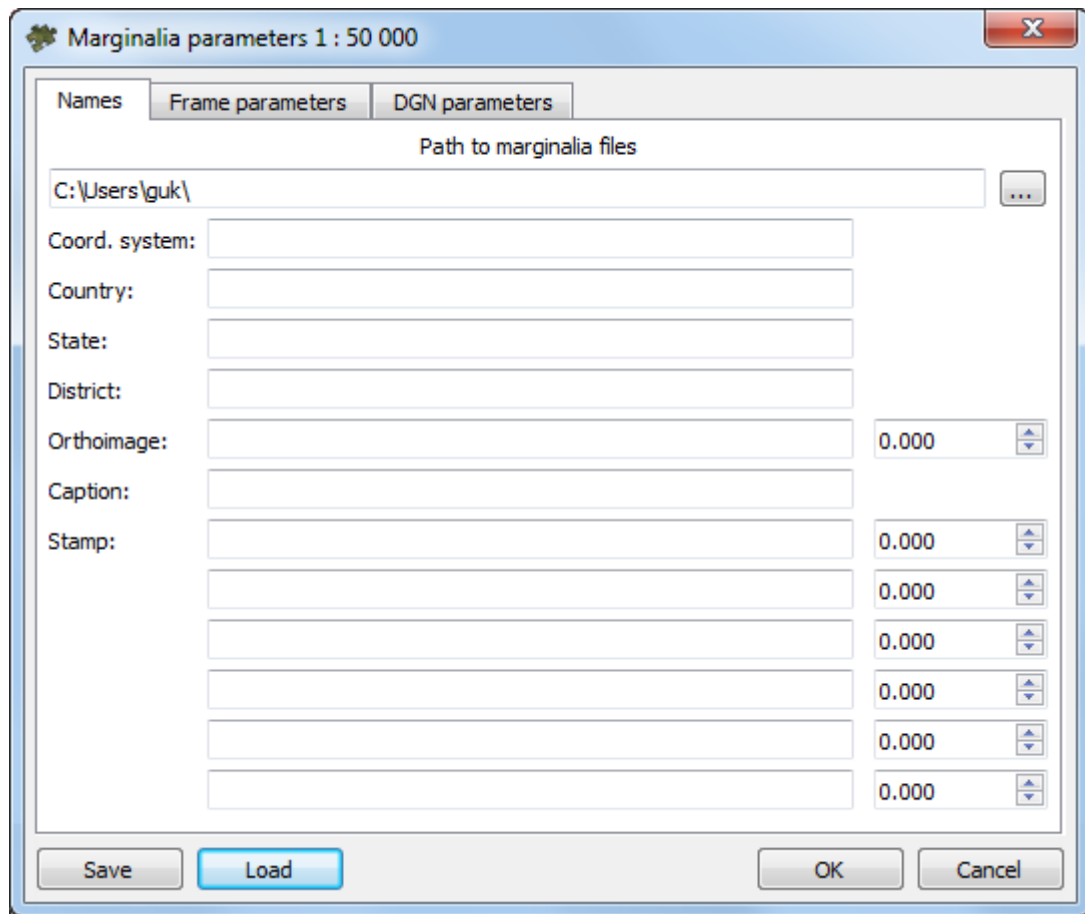
Fig. C.27. Marginalia parameters
