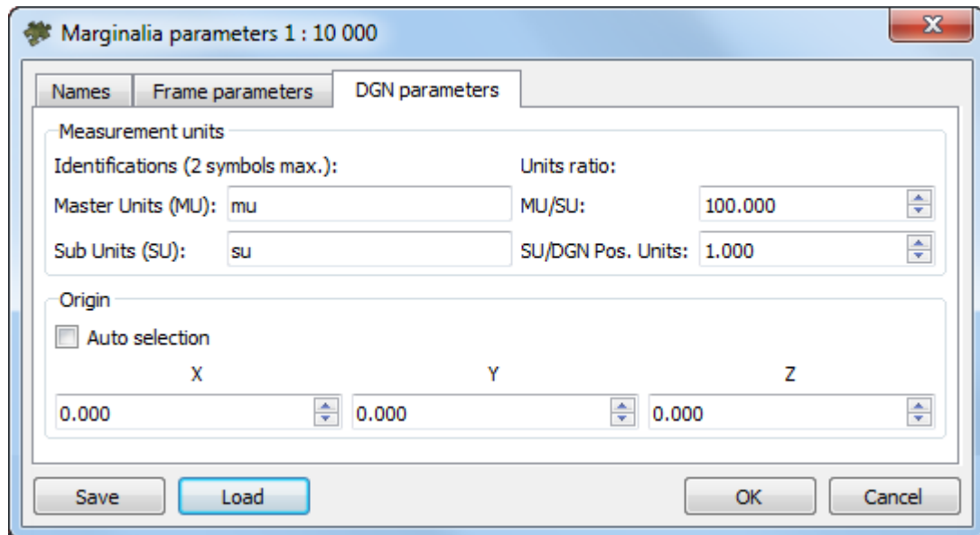
Fig. C.17. Marginalia parameters
