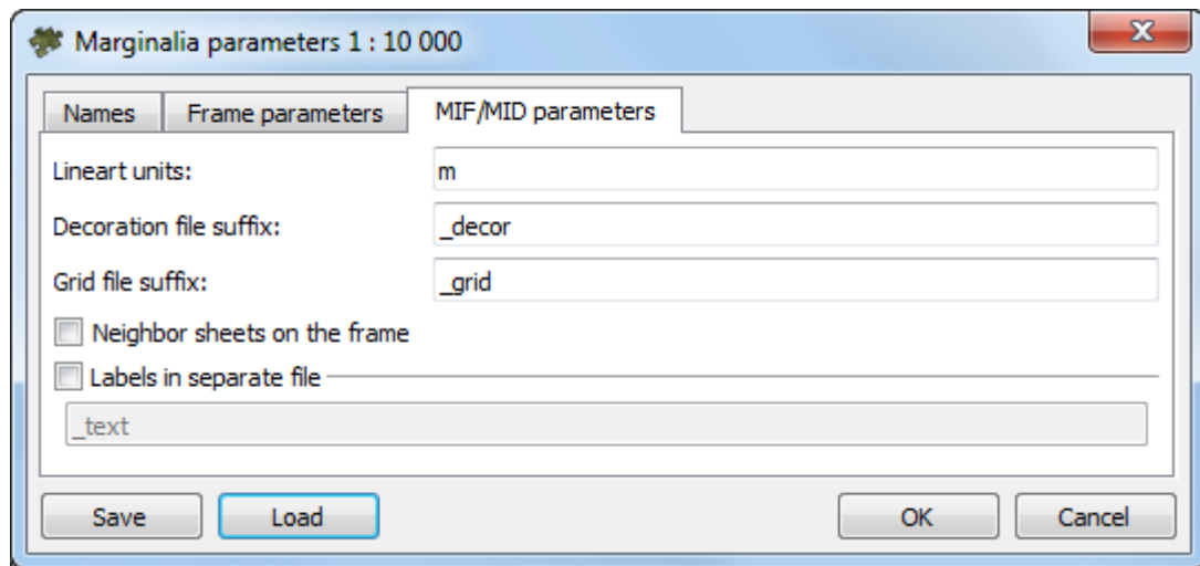
Fig. C.20. Marginalia parameters
