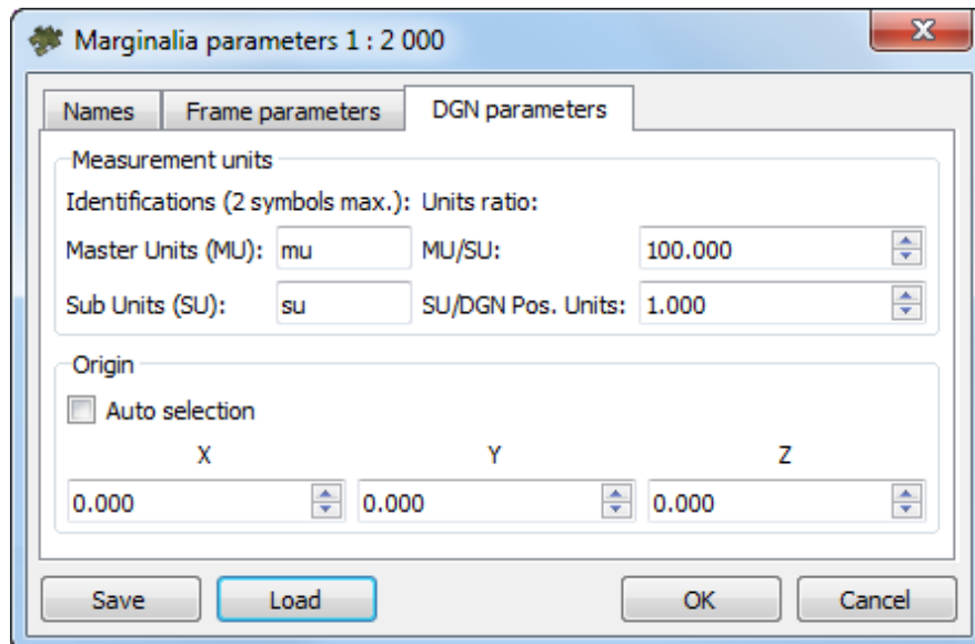
Fig. C.5. Marginalia parameters
