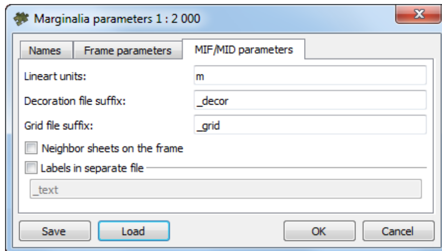
Fig. C.8. Marginalia parameters
