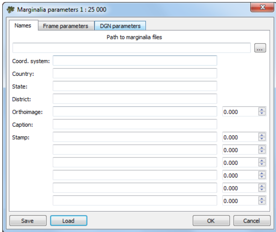
Fig. C.21. Marginalia parameters
