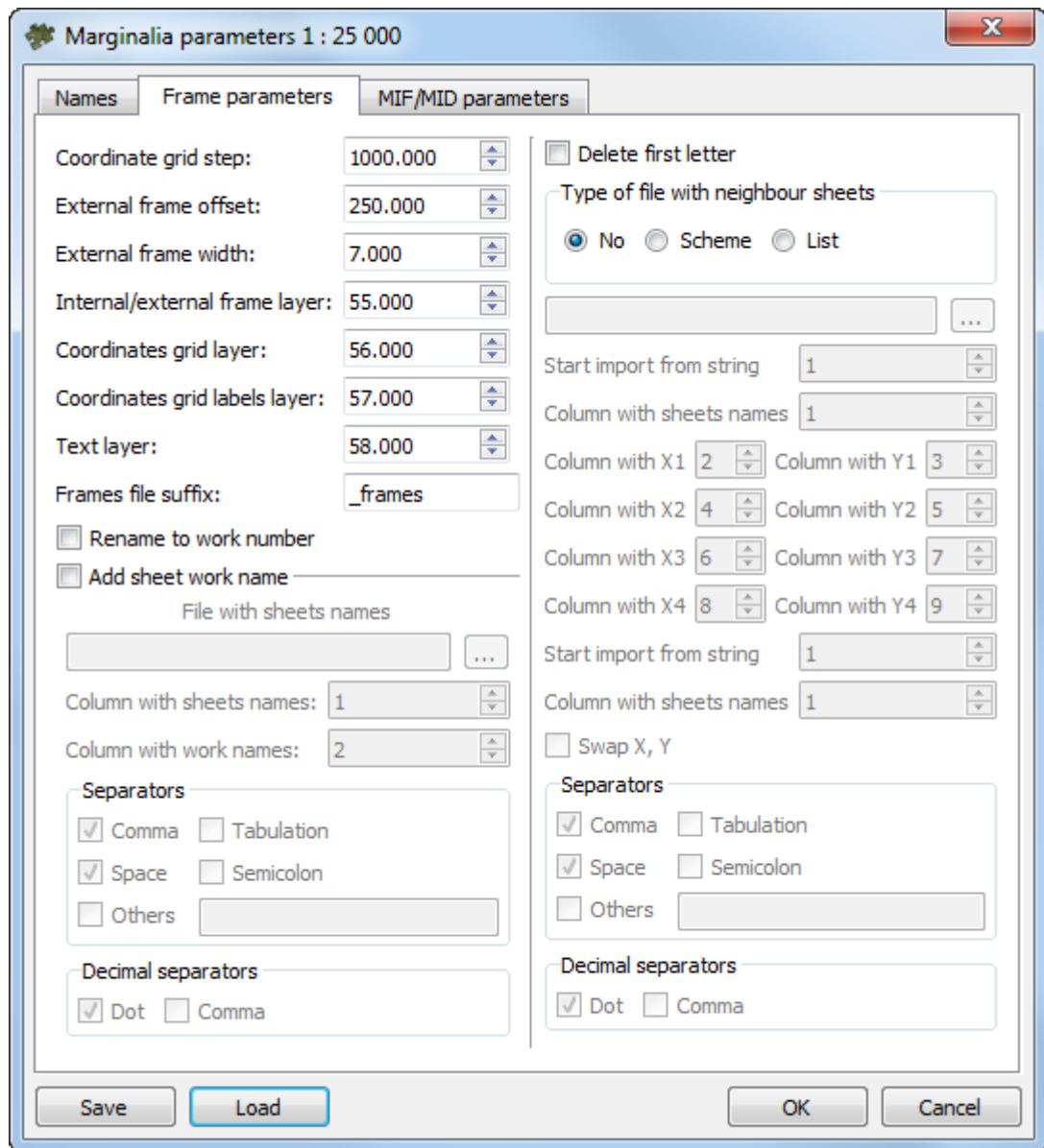
Fig. C.25. Marginalia parameters
