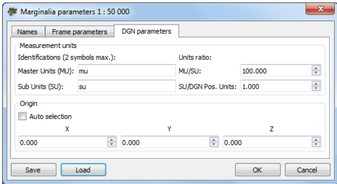
Fig. C.29. Marginalia parameters
