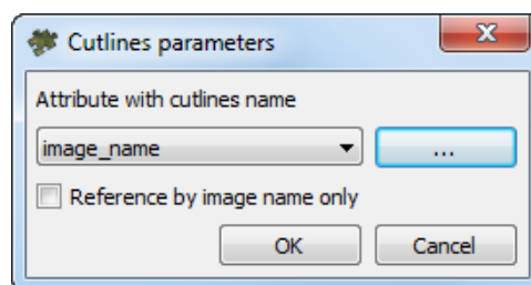
Fig. 26. Cutlines parameters
