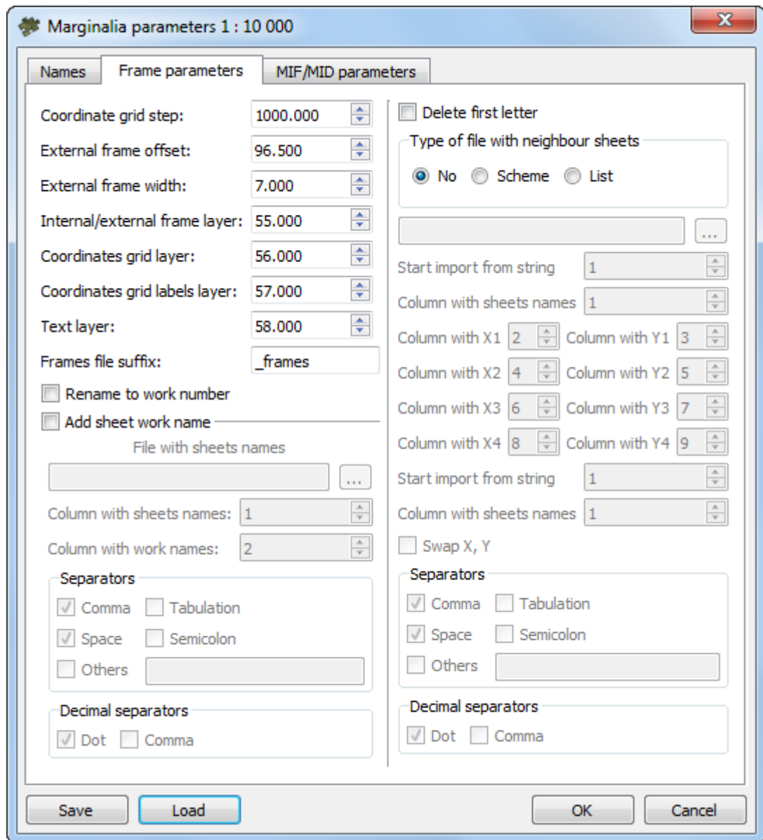
Fig. C.19. Marginalia parameters
