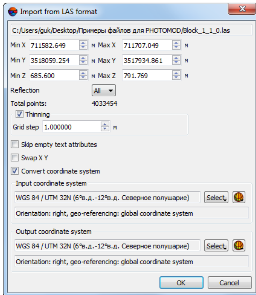
Fig. 227. Import from LAS format
