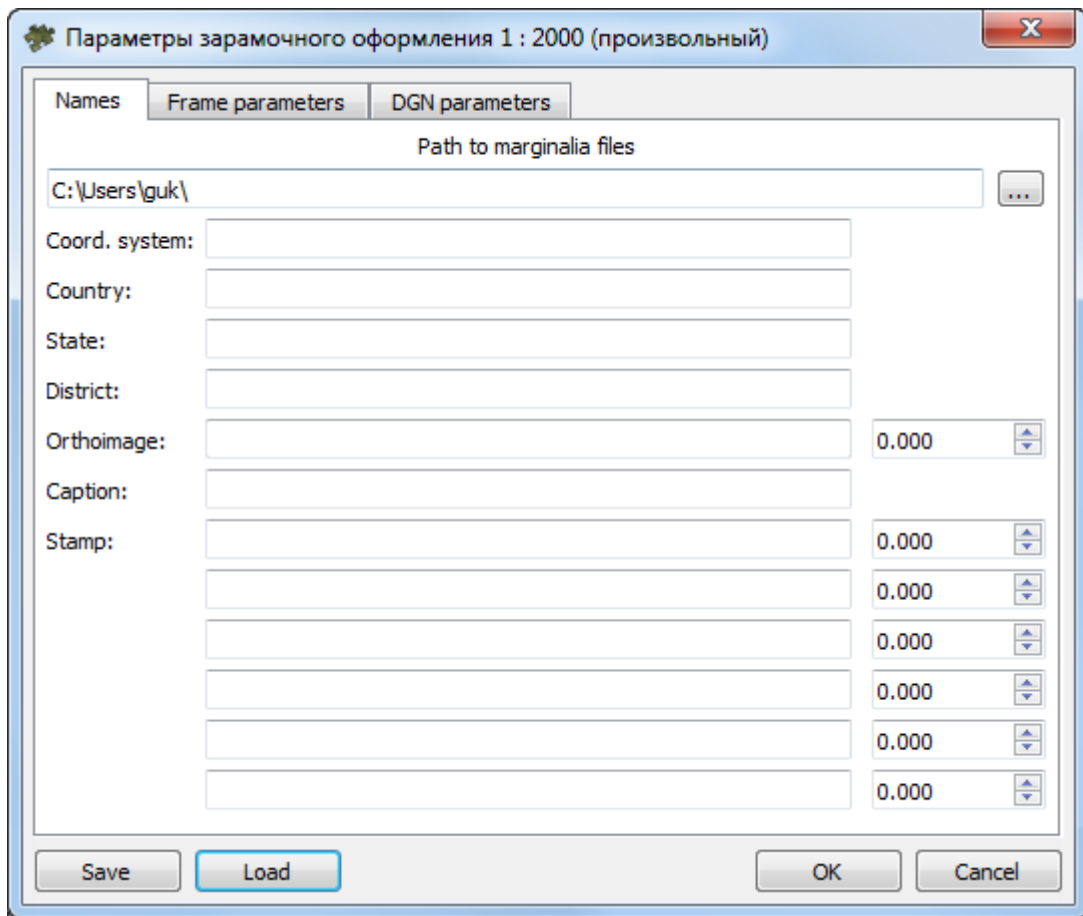
Fig. C.33. Marginalia parameters
