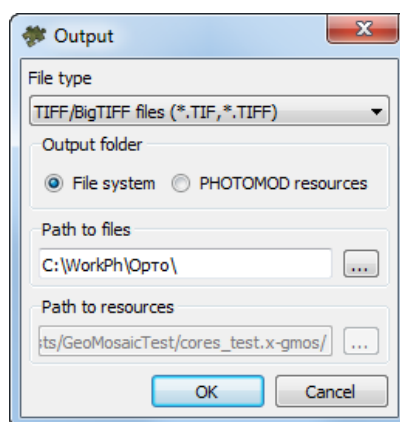
Fig. 71. Output parameters
