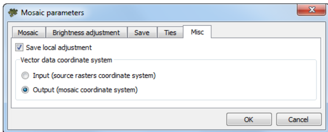
Fig. 70. Additional parameters
